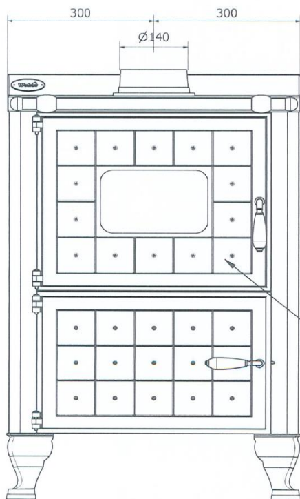
VUE AVANT H 910 mm
