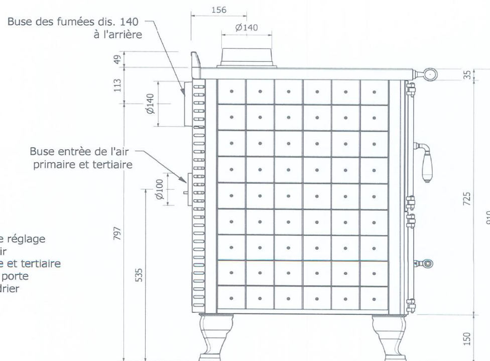
VUE LATÉRALE H 910 mm
